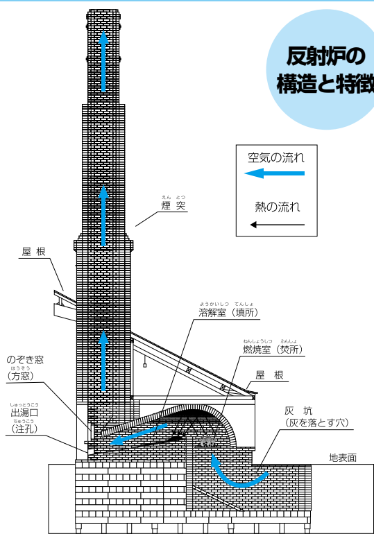
【反射炉断面図】
