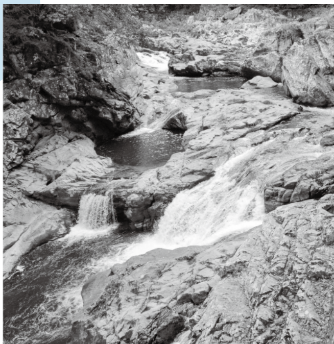
<長門峡(川上～阿東)>古徳佐湖から流出した水(阿武川)が大地を深く削り込んでできた渓谷。運搬された土砂は萩三角州を生んだ。
