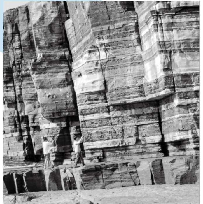
<須佐ホルンフェルス> 日本海が誕生した頃の海底に泥と砂が交互に溜まってできた地層が、マグマの熱で焼きしめられたもの。
