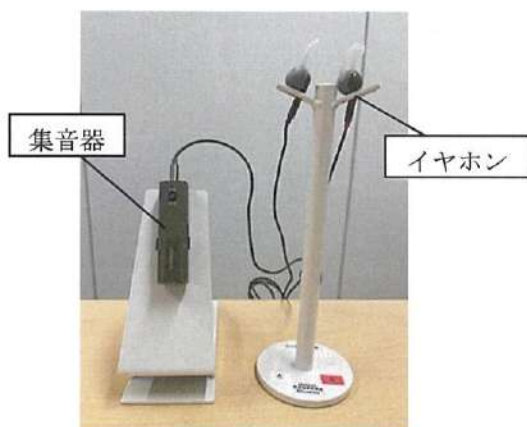
集音器付き軟骨伝導イヤホン
