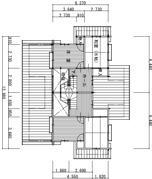
2階平面図 S:1:100
