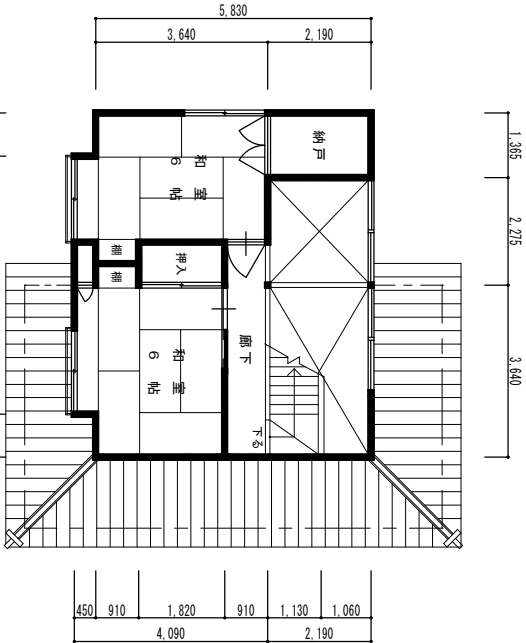
2階平面図
