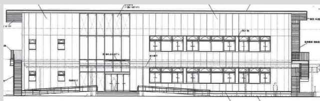
分庁舎南北立面図
