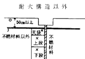
天井裏に感知器がある場合で押入等の壁面が不燃材料のもの
