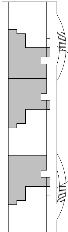
3 階平面図
