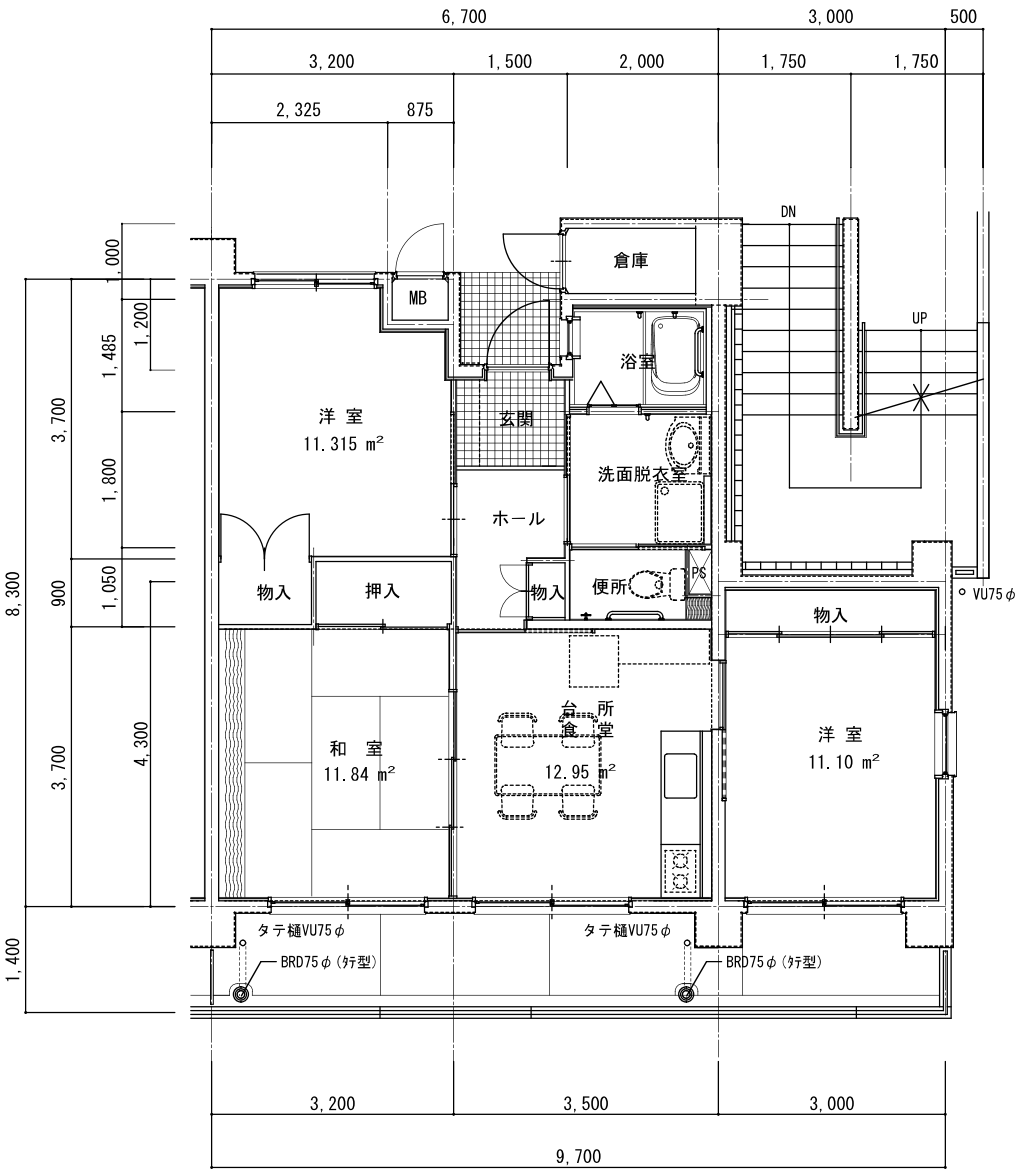
3DK平面図 S=1:100
