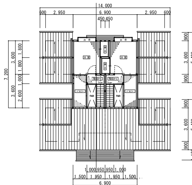
2階平面図 S=1:100
