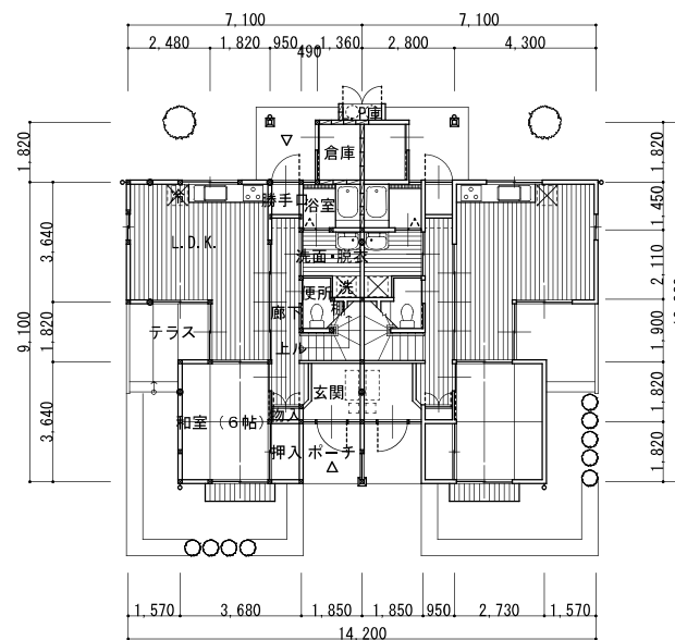
1 階平面図 S. 1:100
