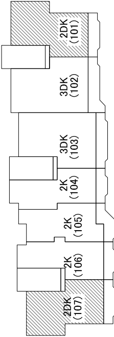
1階平面配置図 S=1:500
