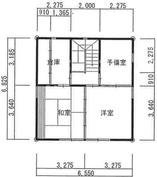
2 階 平 面 図
