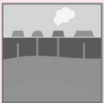
今の萩を作ったマグマの活動
