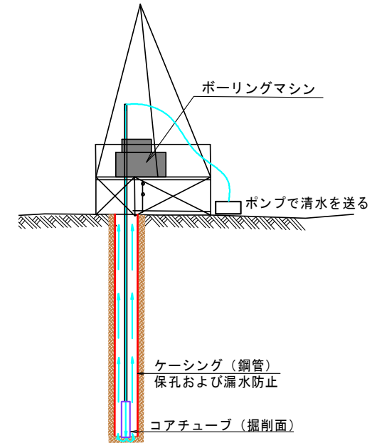
ボーリングに使用するケーシング例
