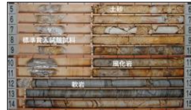
ボーリングで採取したコア例
