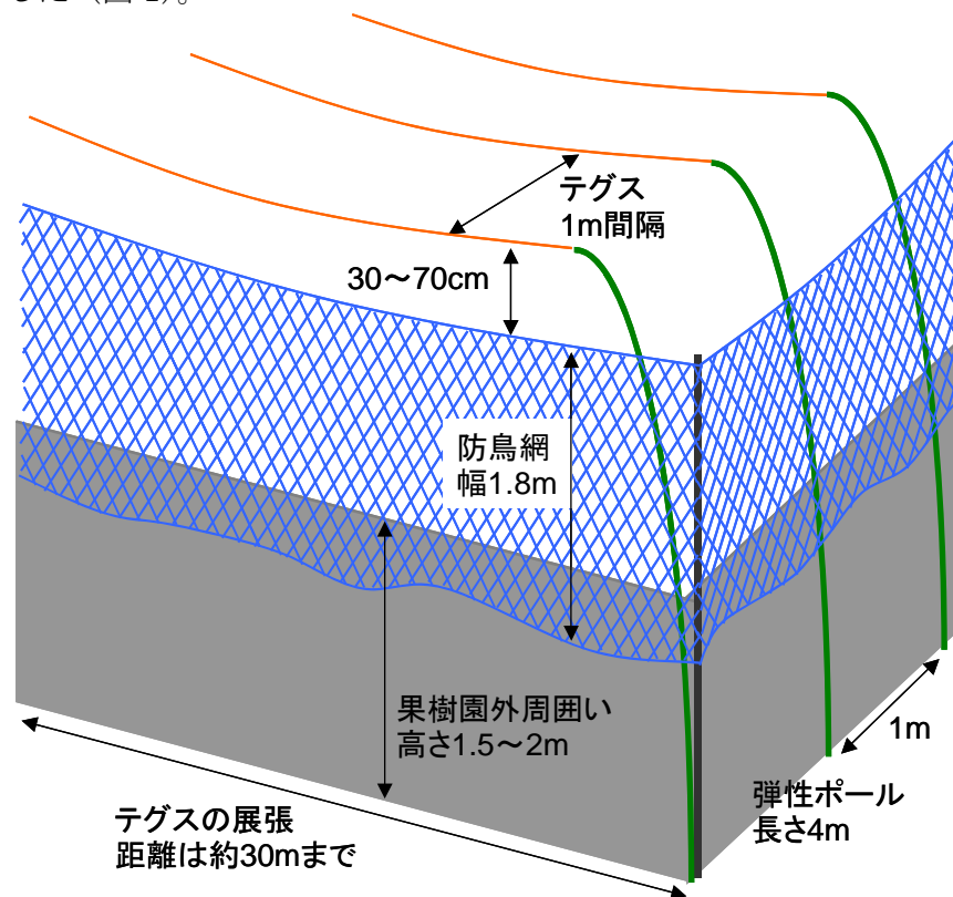
図1 「くぐれんテグス君」の構造見取り図
