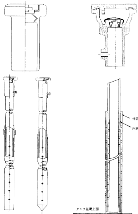
漏えい検査管の管体構造例
