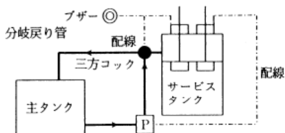
フロートスイッチと分岐戻り管等
