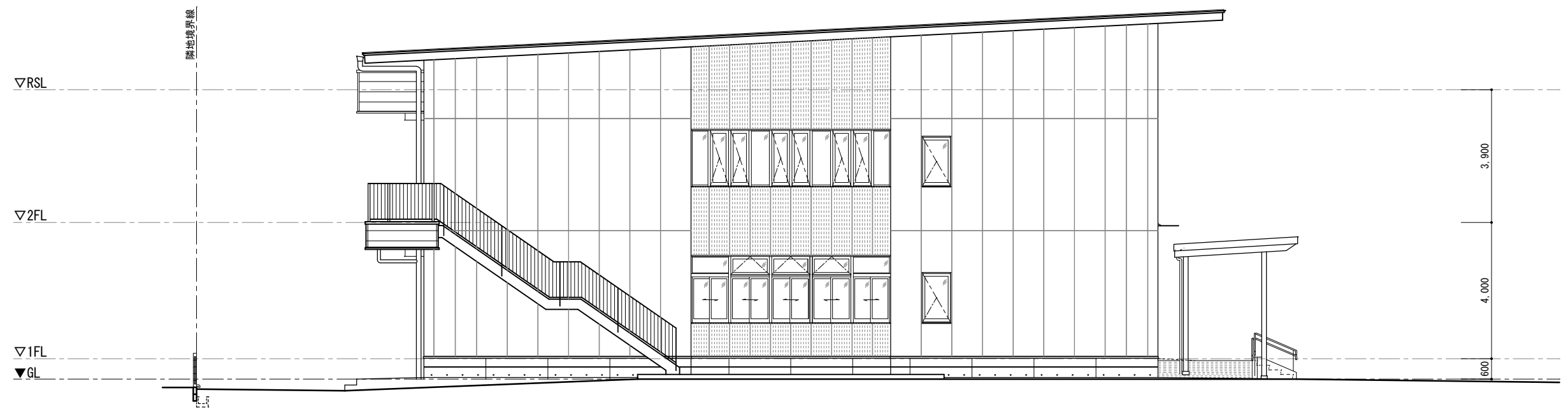
東立面图 S=1/100
