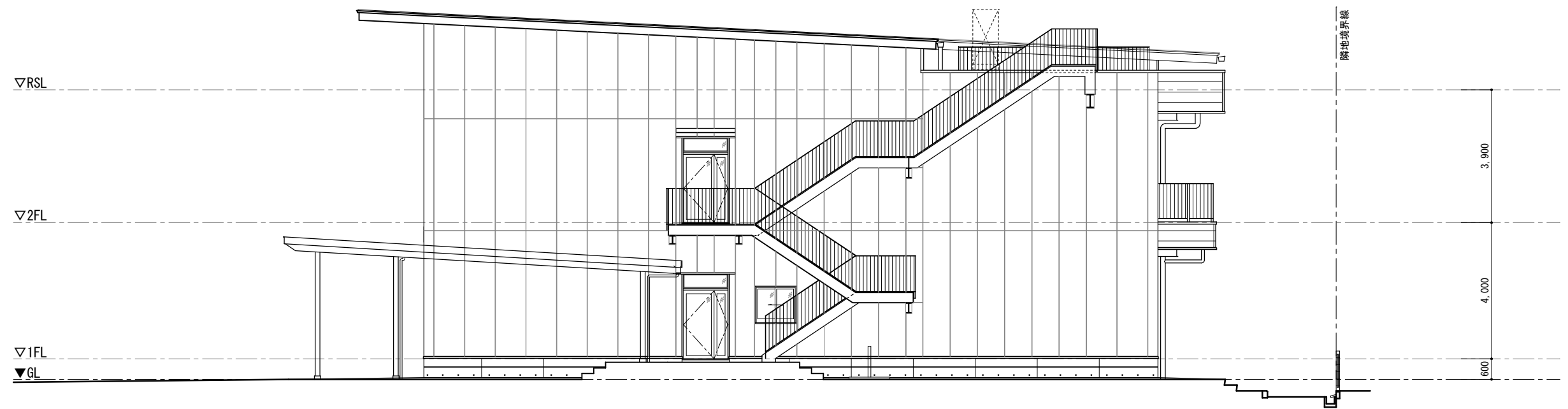
西立面图 S=1/100
