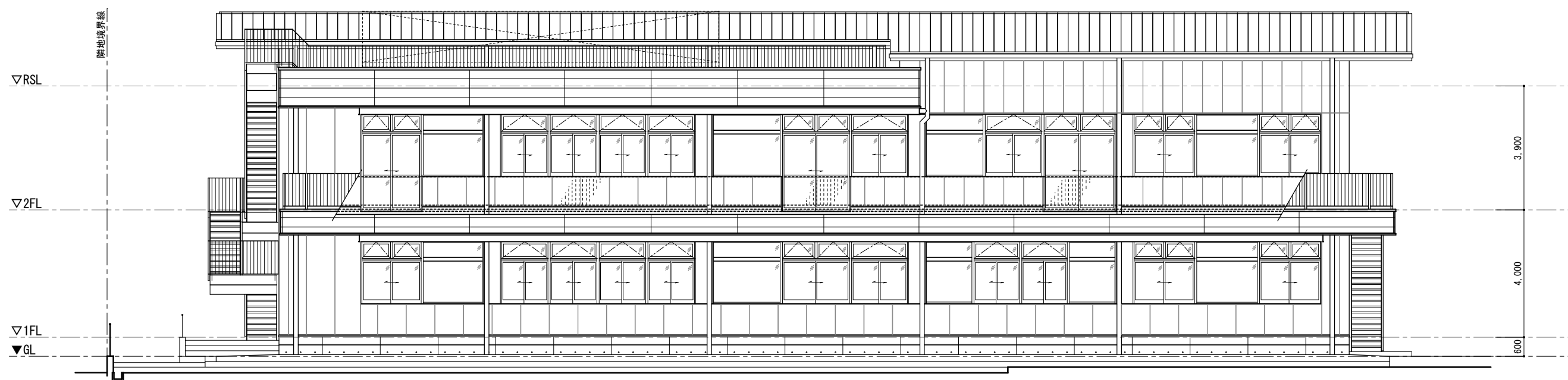
南立面图 S=1/100
