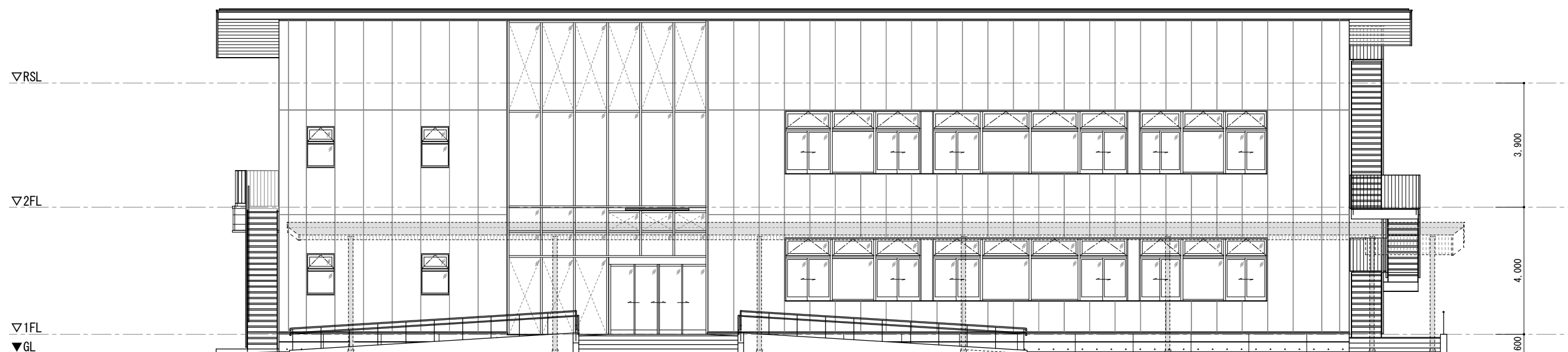
北立面图 S=1/100
