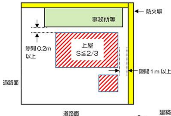
・認められる例1 (平面)
