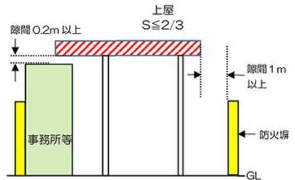
・認められる例2 (立面)
